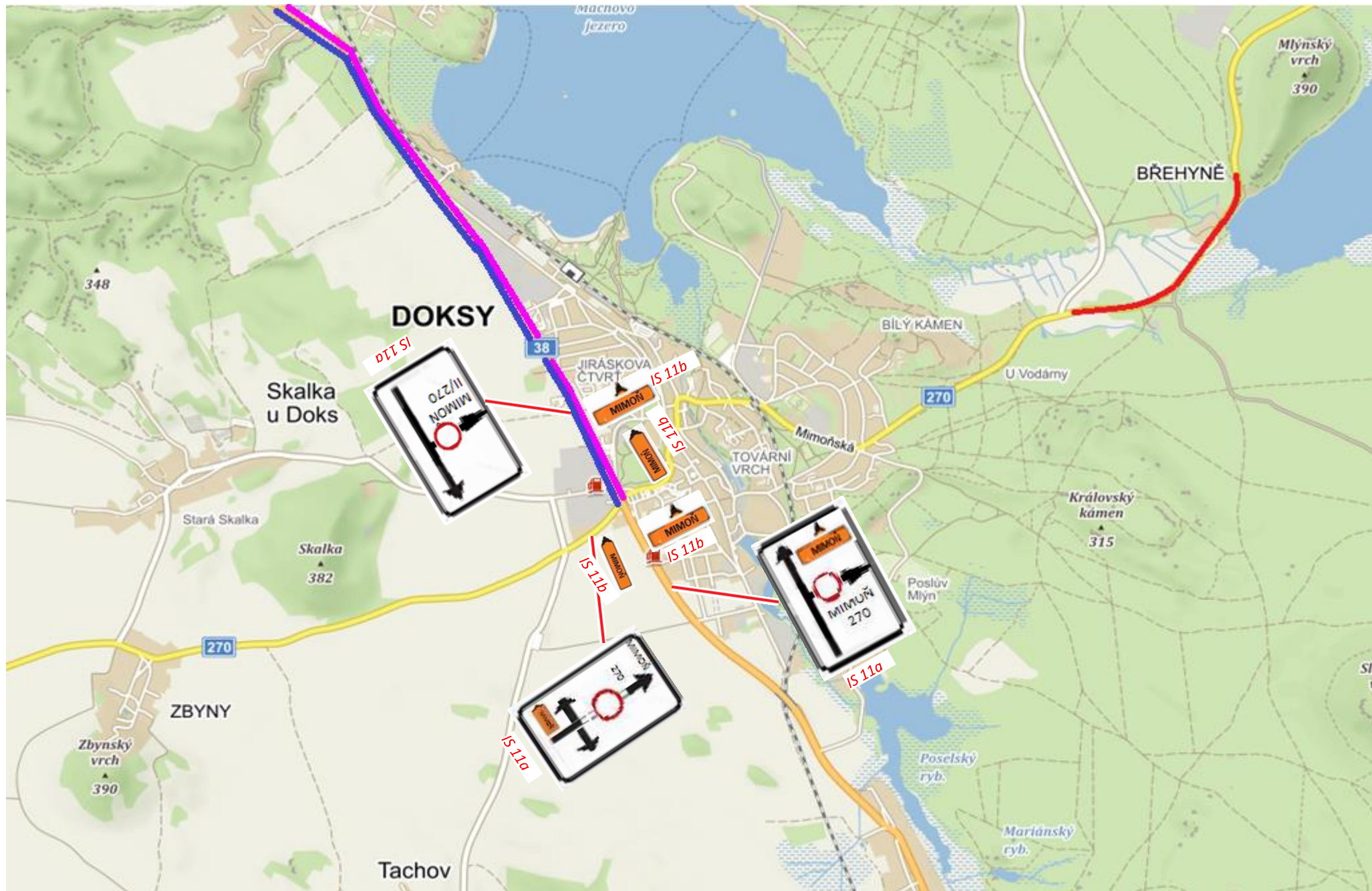
DIO – Detail č. 1 – křiž. sil. I/38 a II/270 - Doksy
