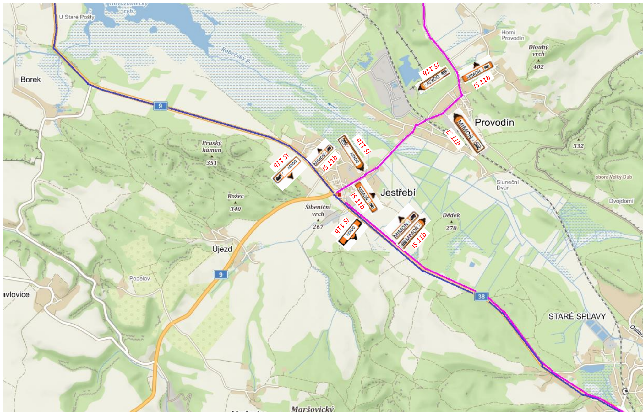
DIO – Detail č. 2 – JESTŘEBÍ – křiž. sil. I/9, I/38 a III/26832
